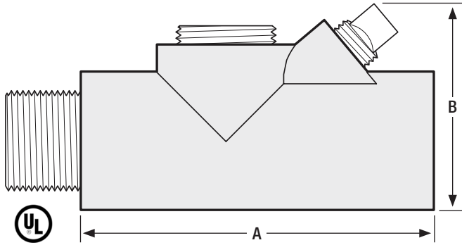
Conduit seal dimensions
