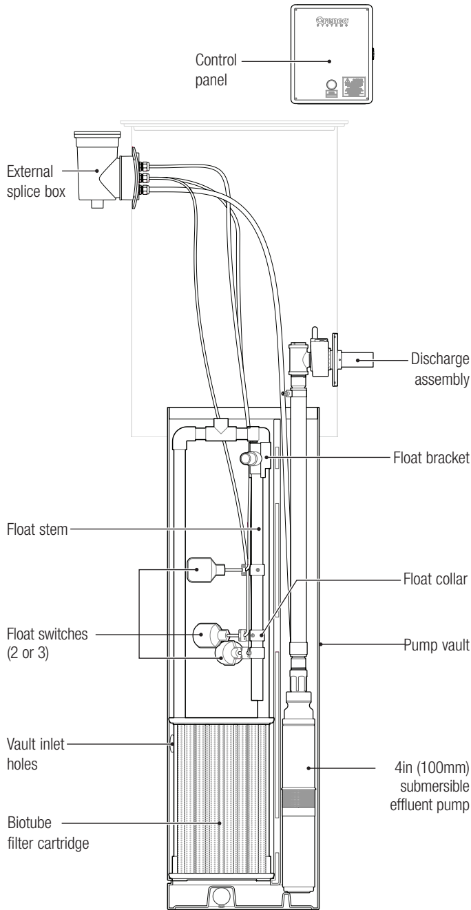
Biotube 60Hz LOS Pump Package
